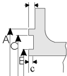
Type D Groove face
